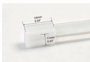
End cap
